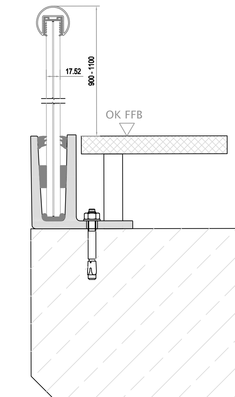
Bodenverschraubung
