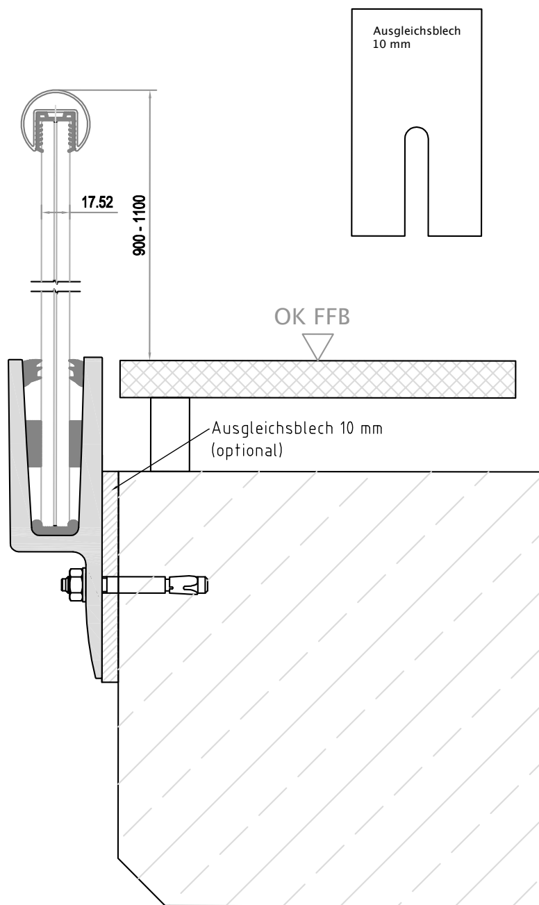
Vorwandverschraubung
